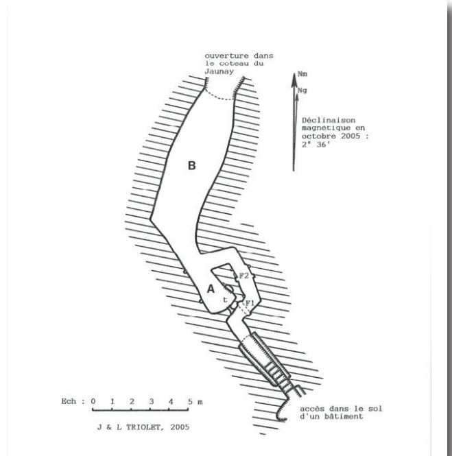
Plan du souterrain-refuge à défense active de la Gillaudière (plan J. & L. Triolet 2005).
